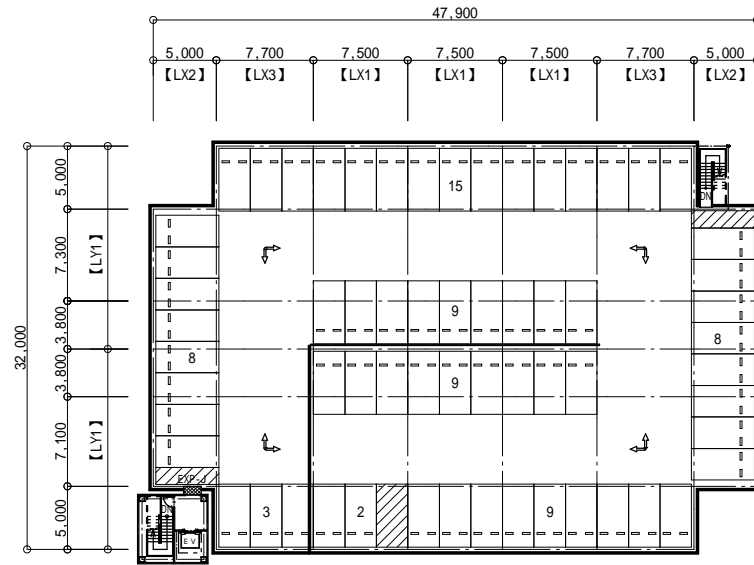
R階 平面図
