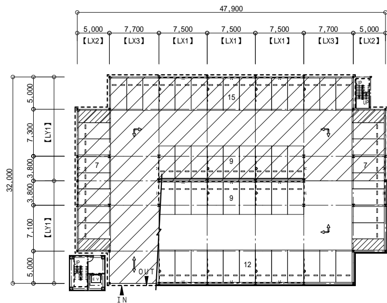
1階 平面図
