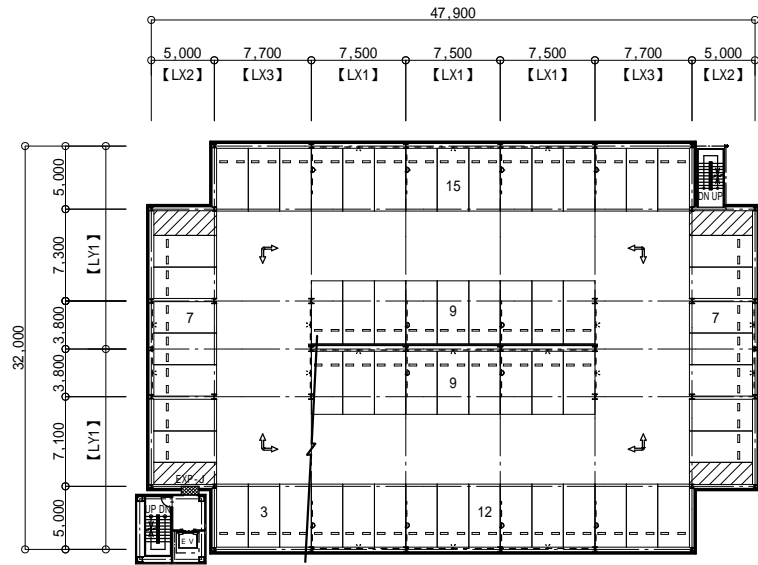
2 ~ 4階 平面図
